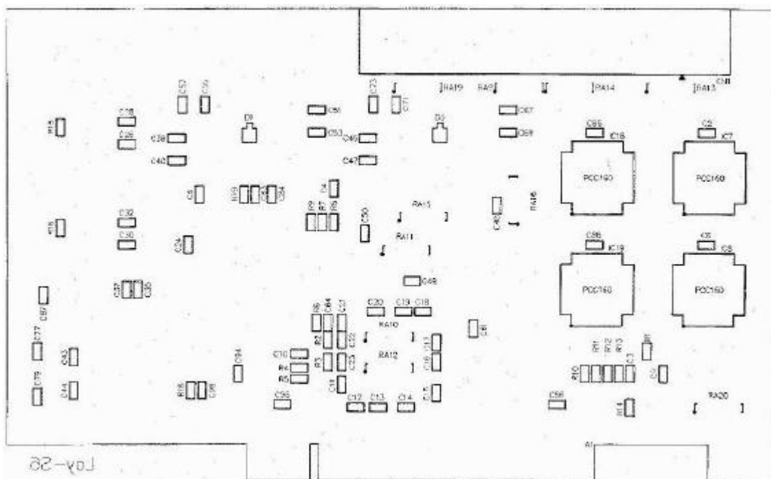
ポート裏の部品配置
